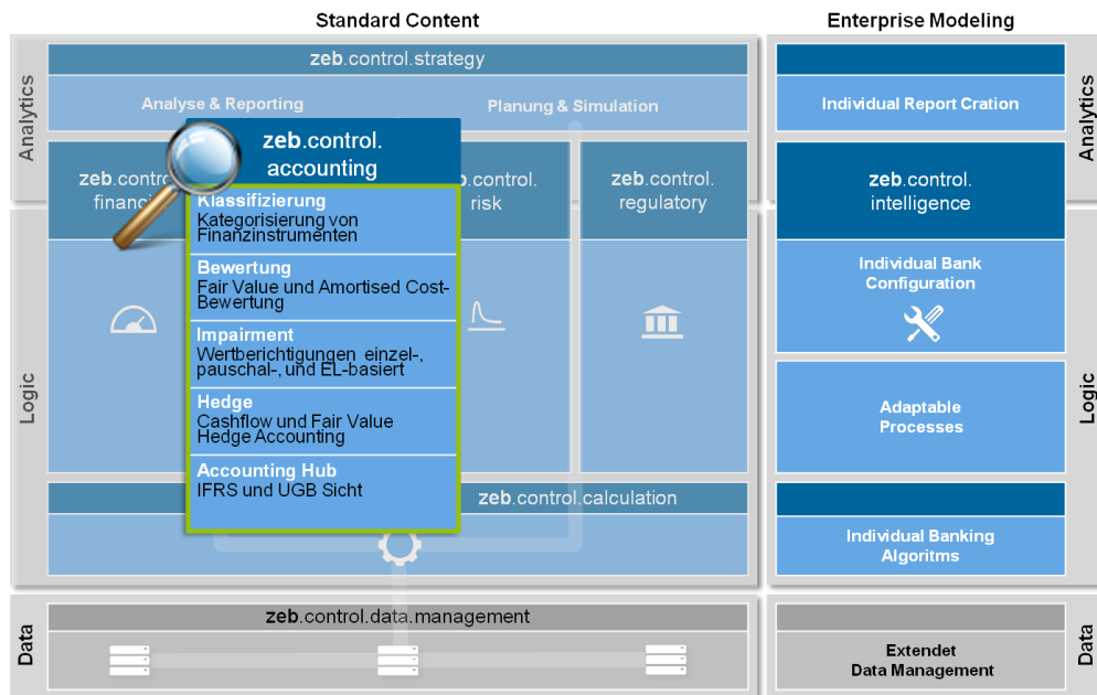
Abbildung 1: Architektur zeb.control.accounting
