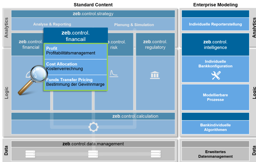
Abbildung 1: Architektur zeb.control.financial
